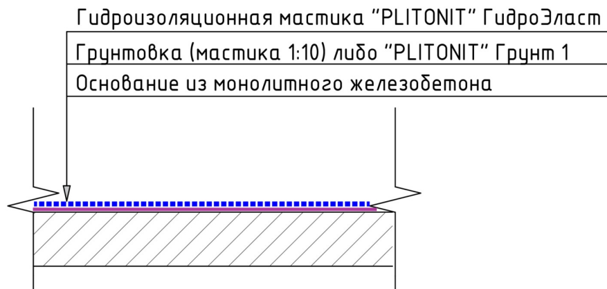
Сечение готового покрытия гидроизоляции.
